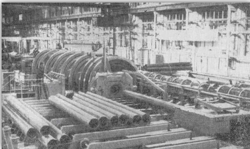
Трубоволокательный стан кольчугинского завода им. С. Орджоникидзе – гигантский механизм, выпускающий трубы различных размеров
